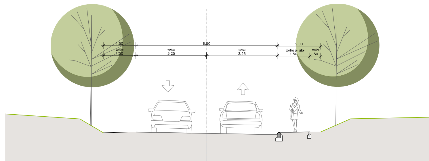
Prečni prerez nove dostopne ceste v UE-02
